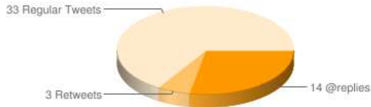
Tweet Types
